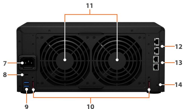
Задняя панель
