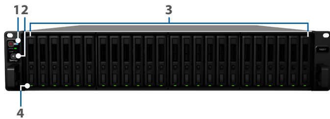
Передняя панель
