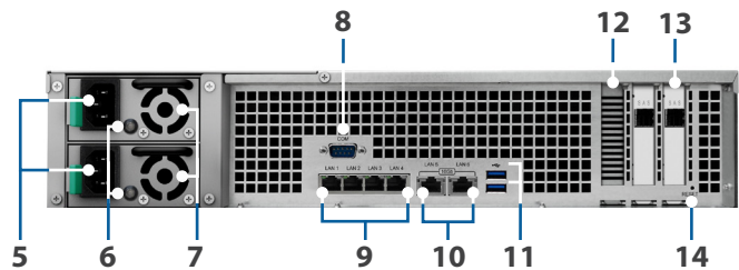
Задняя панель
