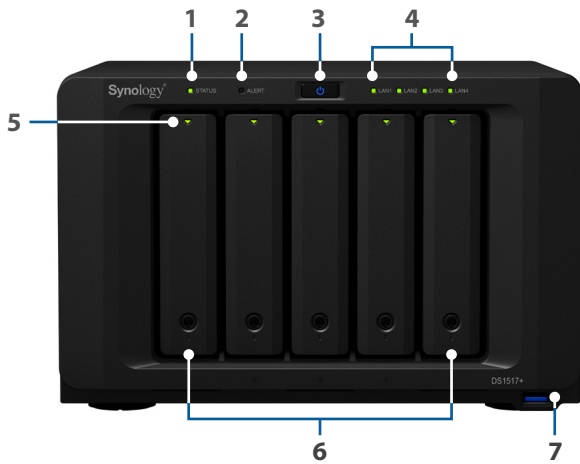
Передняя панель
