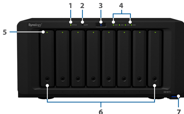
Передняя панель
